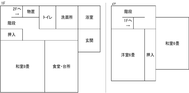
【薬師住宅】
