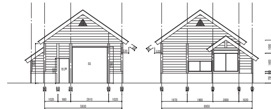
東側立面図 S=1:200
