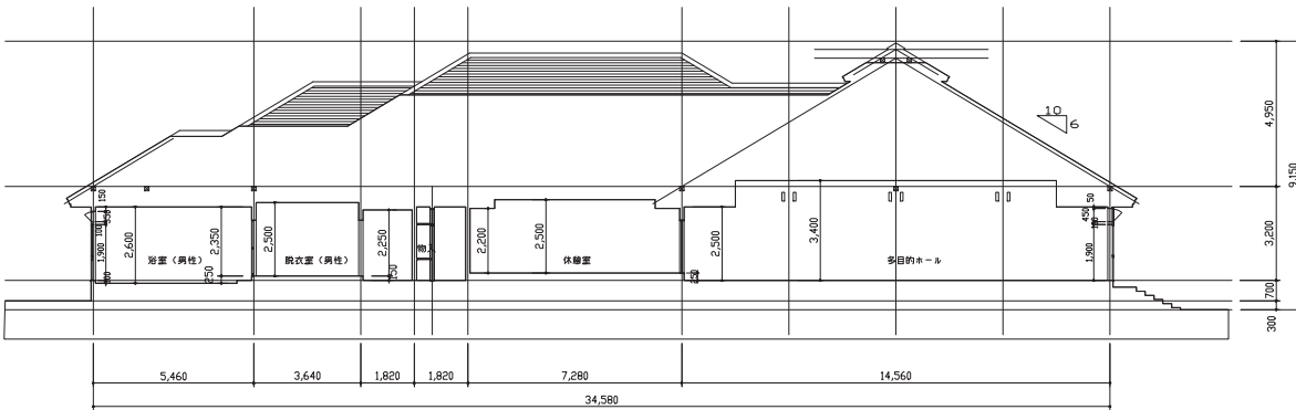
断面図 S=1:200
