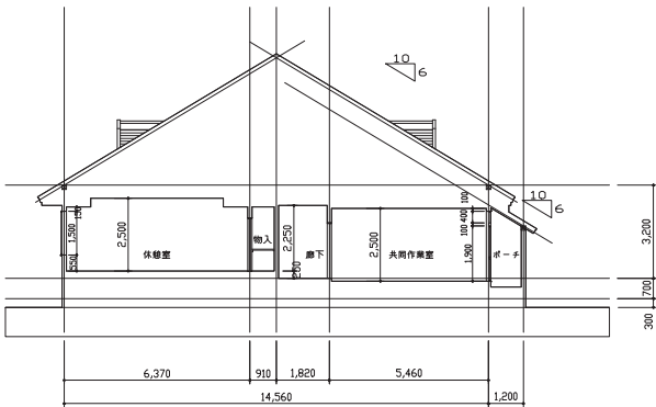
断面図 S=1:200
