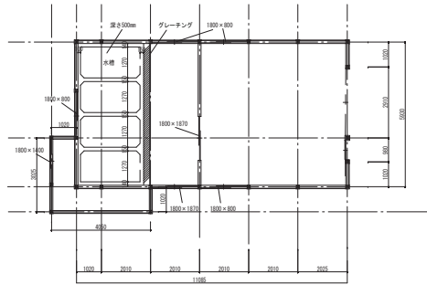
平面図 S=1:200
