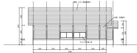
北側立面図 S=1:200
