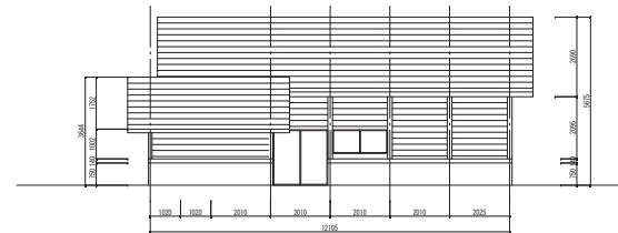
南側立面図 S=1:200
