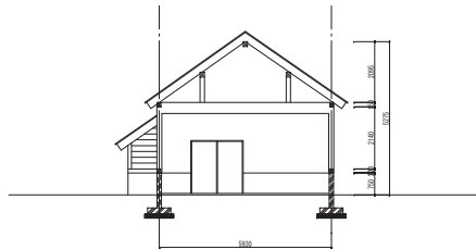
断面図 S=1:200
