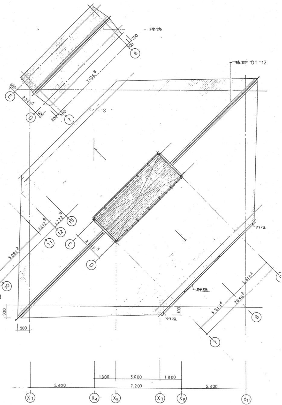
屋根伏図
