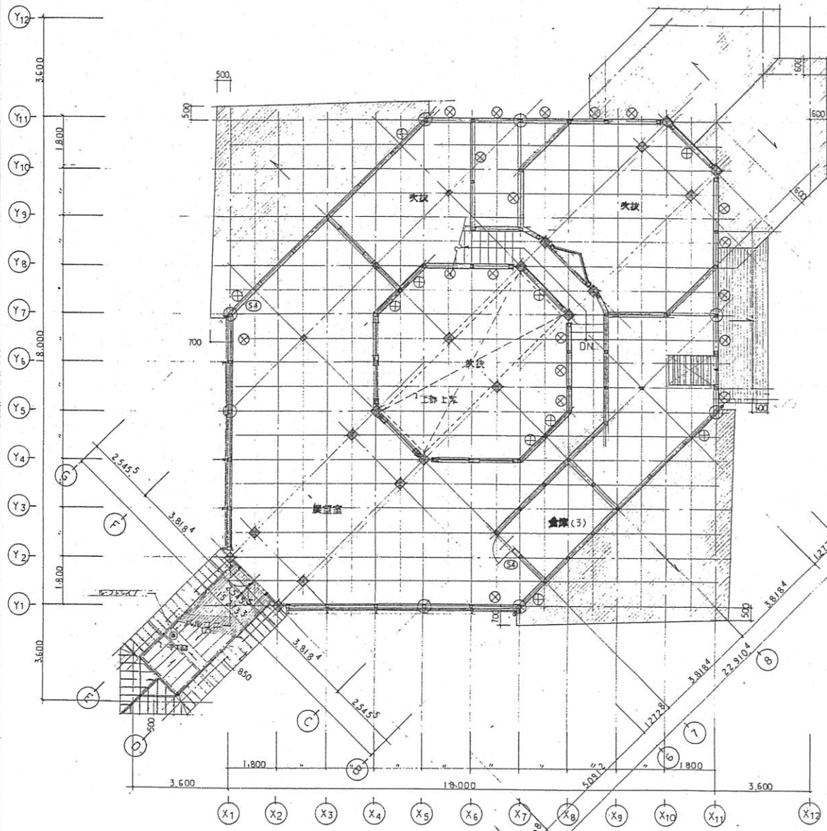
2階平面図
