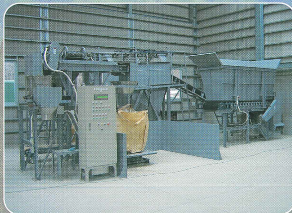
選別袋詰装置
