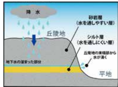
▲高清水湧水のしくみ
