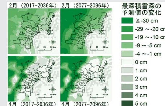
図2 地域気候モデルによる近未来(2017～2036年)、21世紀末(2077～2096年)における宮城県2月と4月の最深積雪の予測値の変化
